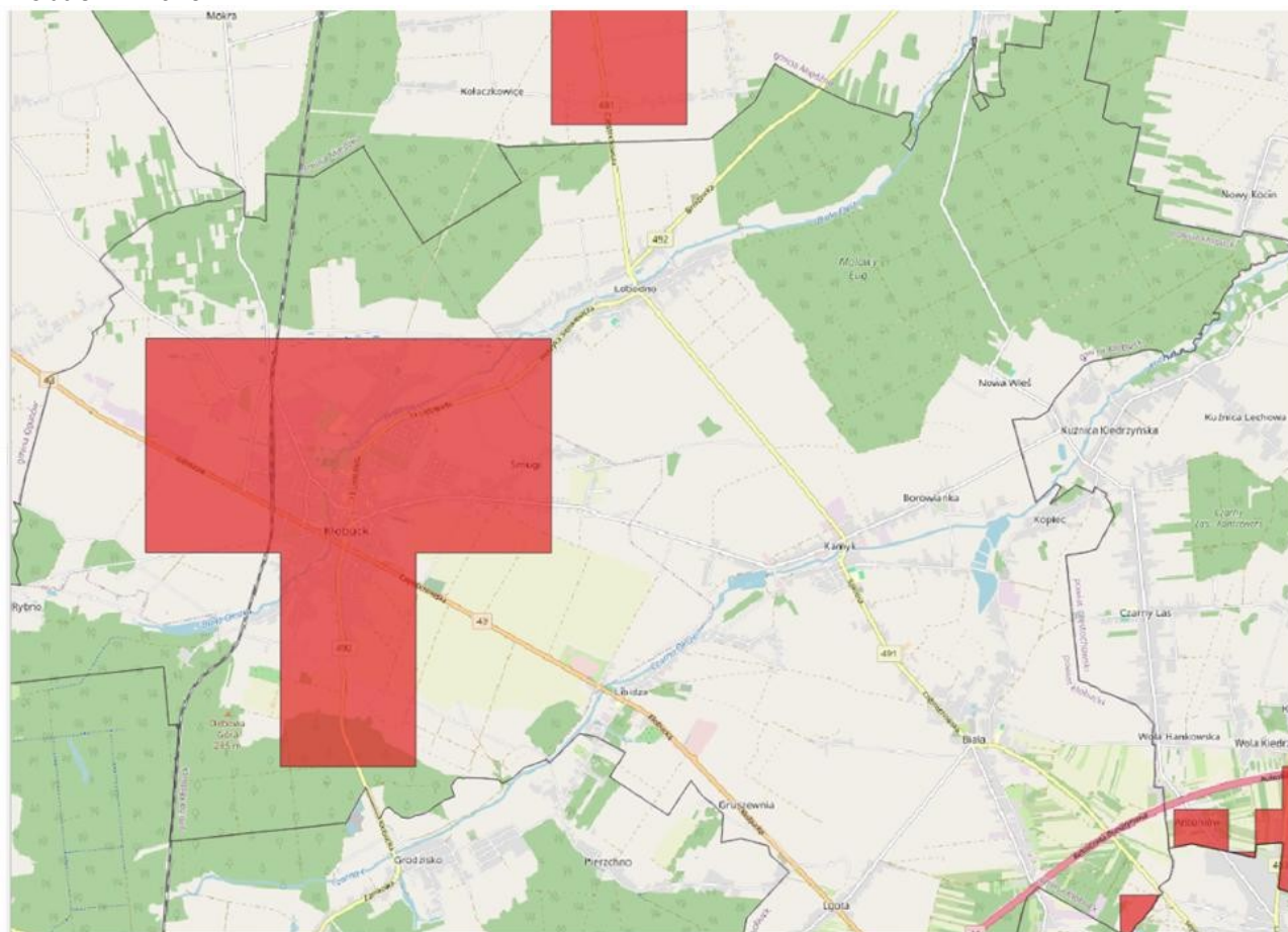
Rysunek 10. Zasięg obszaru przekroczenia poziomu docelowego B(a)P na obszarze gminy Kłobuck w 2025 r.
